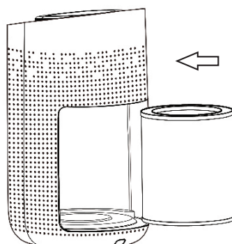
⑤ Sätt i det nya HEPA-filtret i 49200. Den öppna sidan uppåt
