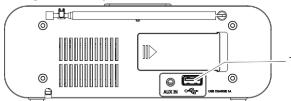
Figure 4 : Connexion USB pour charger des appareils externes
