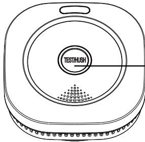
Test / Stummschalt-Taste
